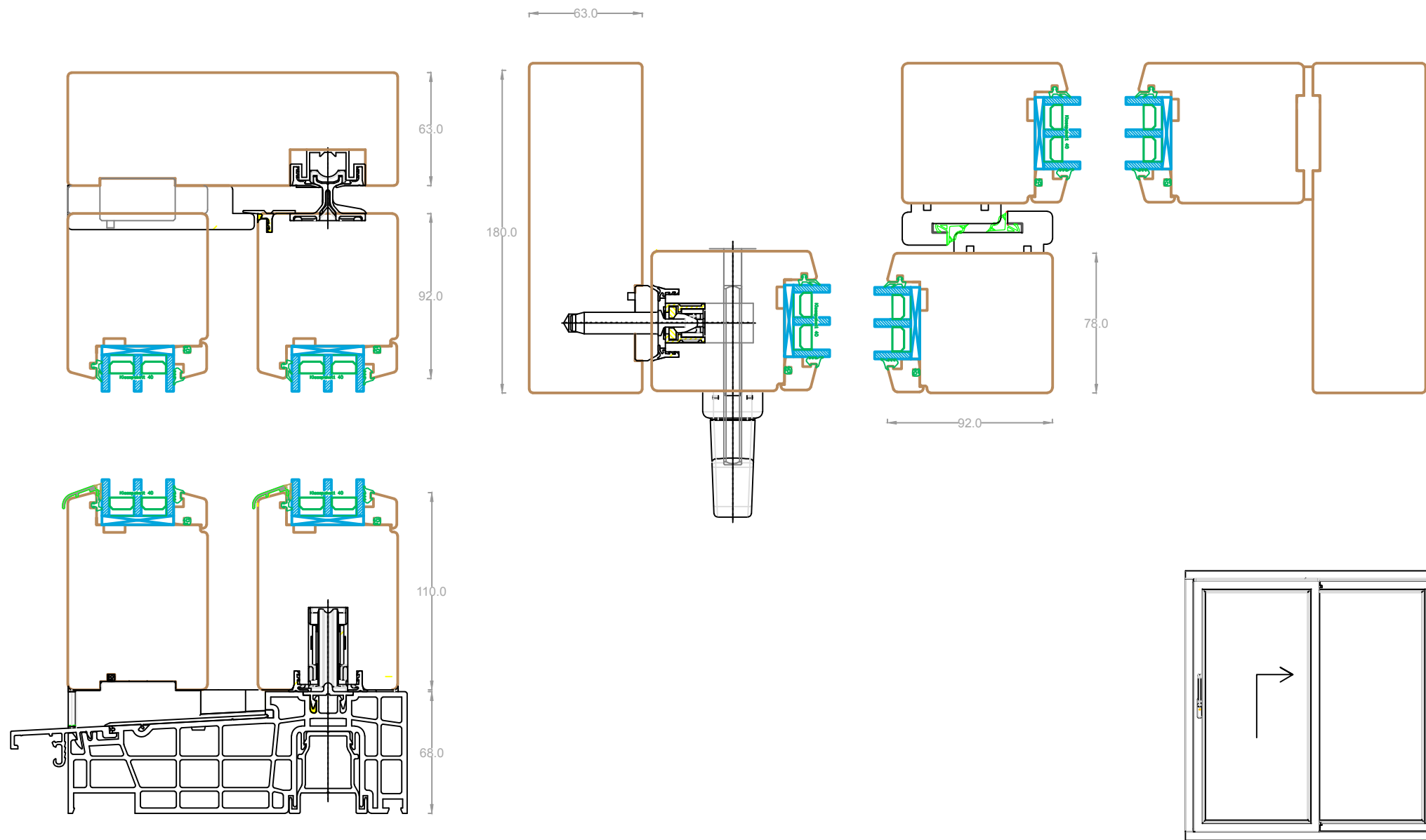
Tõst-lükanduks GU78, skeem A
