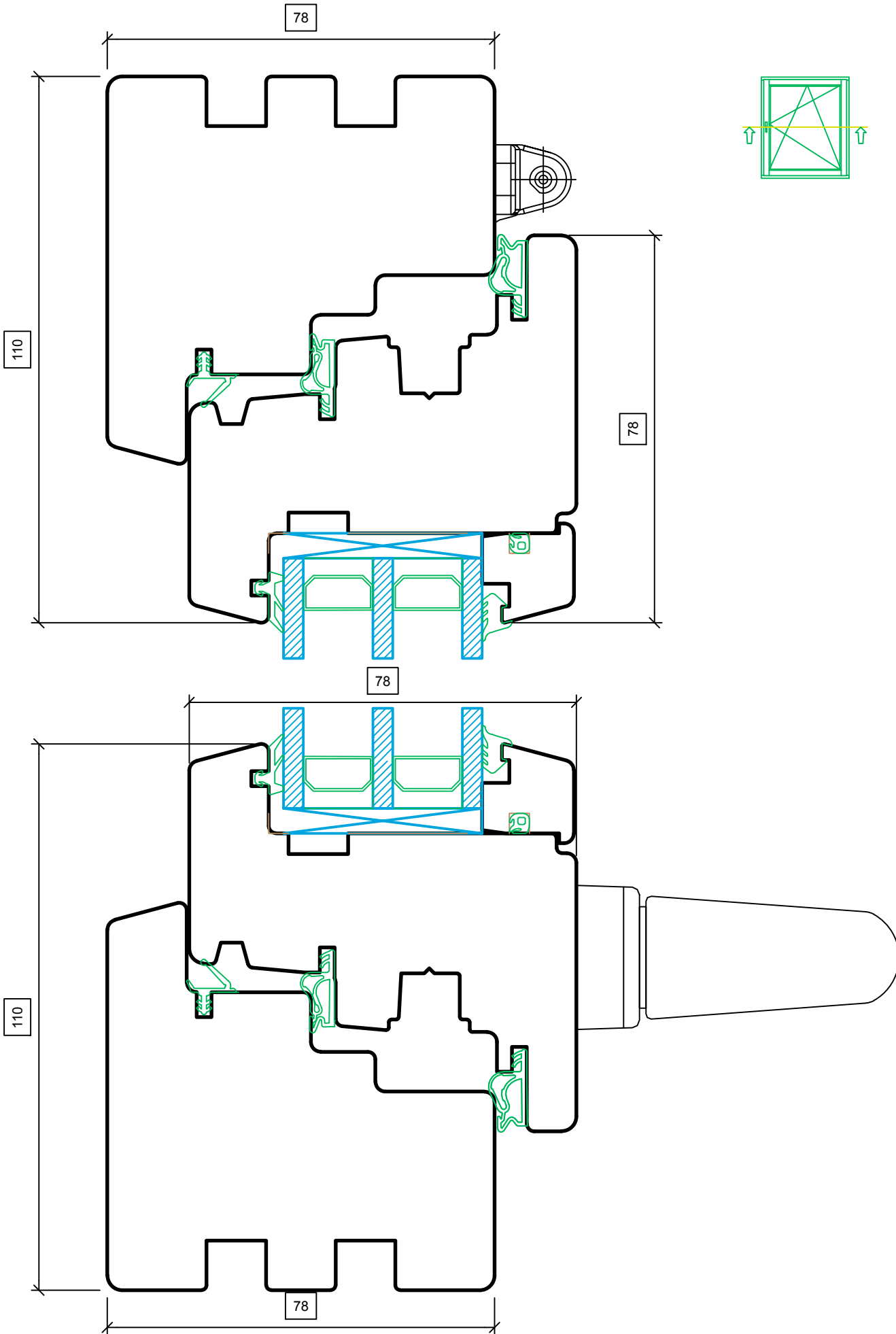
Sisepoole avatav rõduuks IV78 madala lävepakuga Horisontaalne ristlõige * Tootja jätab endale õiguse teha muudatusi.
